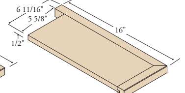
K-8071-2RE18 5-5/8" x 11-1/2" Specify LH or RH (RH Shown)
